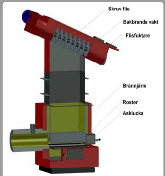
Flisbrännare 04E i genomskärning.
